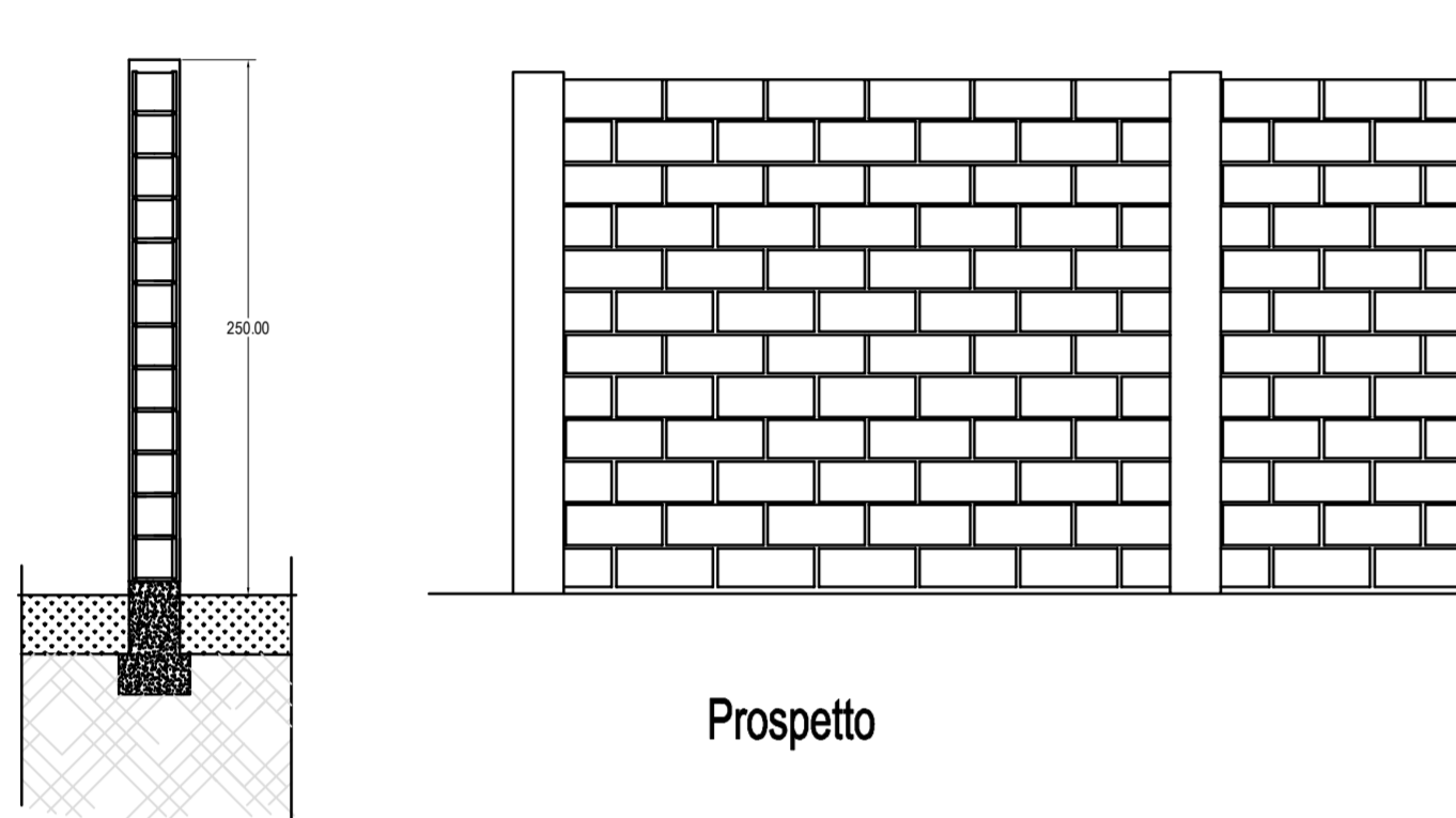
recinzione tra i lotti - sola Muratura a vista o intonaco civile
